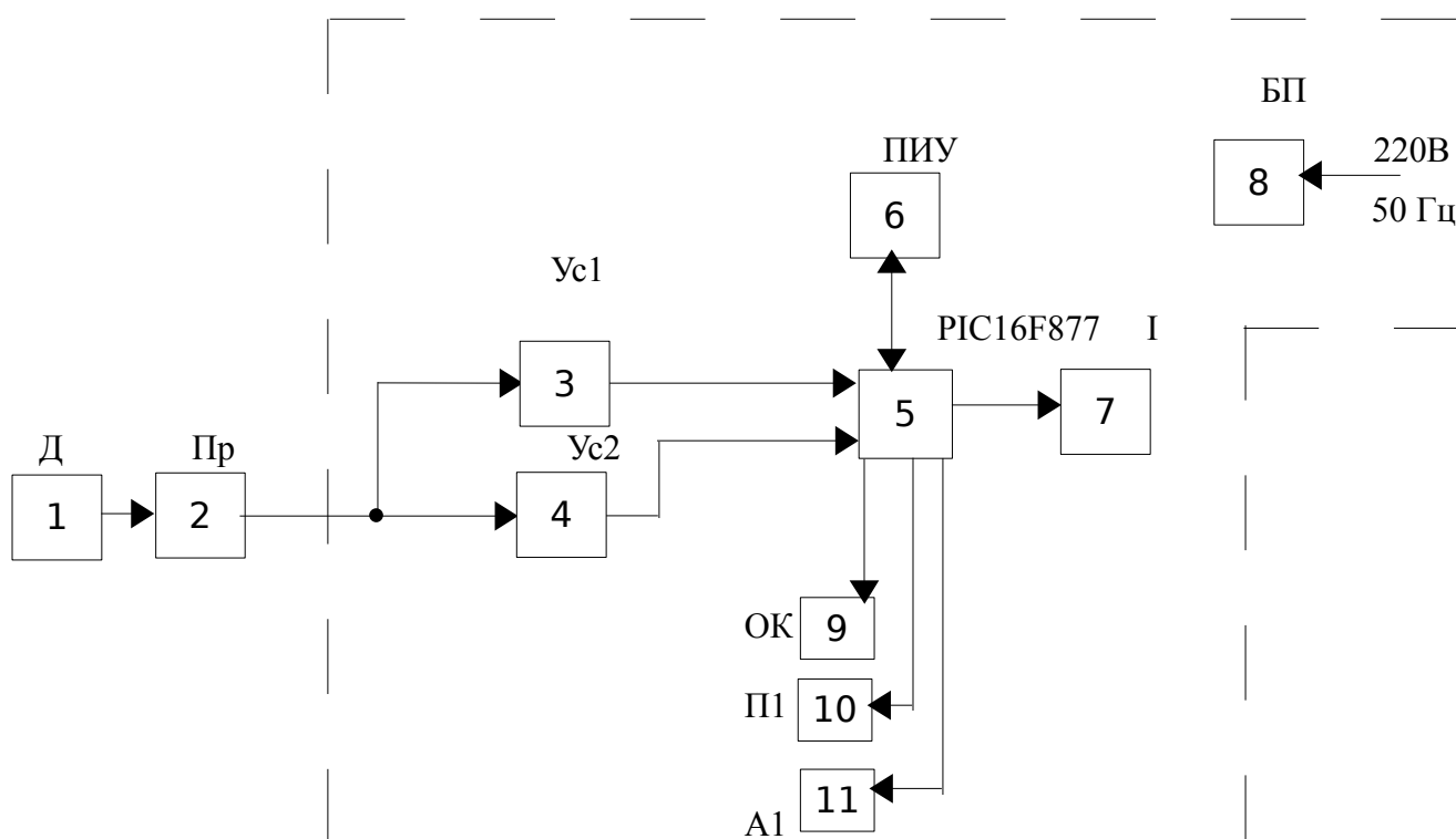
Структурная схема устройства ИП-106.
